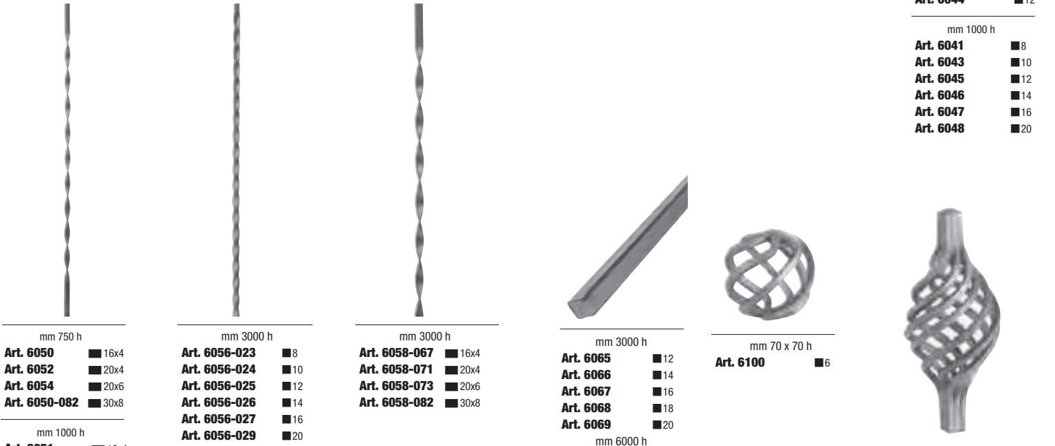
Art. 6110 ■ 12 mm 65 x 125 h Art. 6112 ■ 15 mm 70 x 150 h Art. 6114 ■ 21 mm 85 x 170 h Art. 6116 ■ 24 mm 95 x 220 h Art. 6118 ■ 30 mm 95 x 240 h
